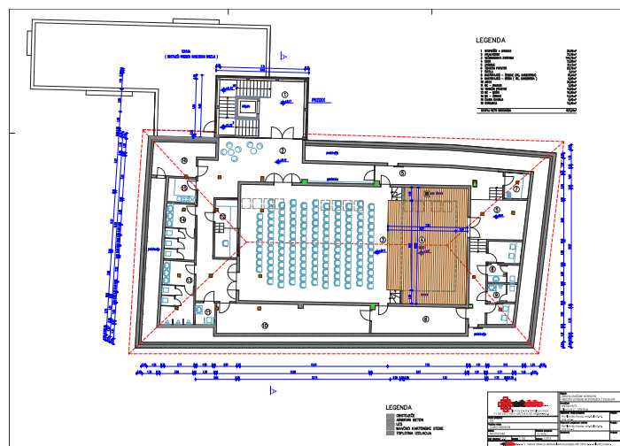
Slika 2: Idejna zasnova ureditve mansarde za večnamensko dvorano
